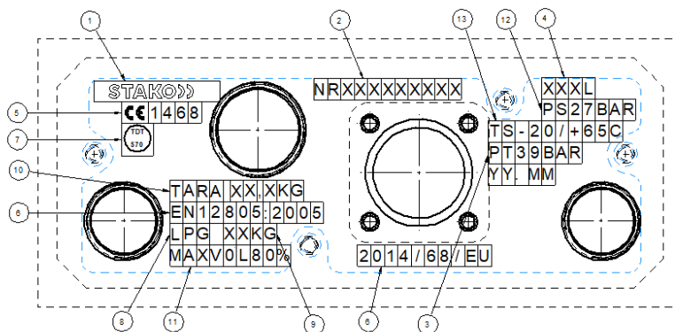
Rysunek 2. Zawartość tabliczki znamionowej zbiornika LPG
